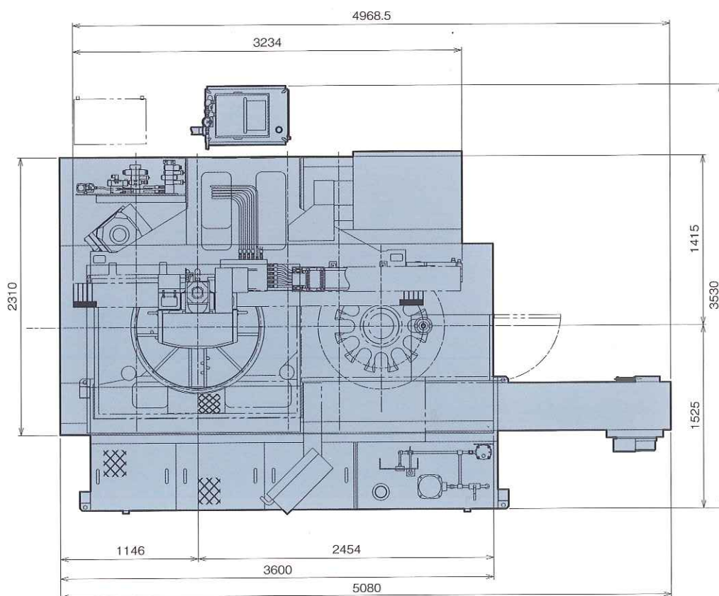
平面図
